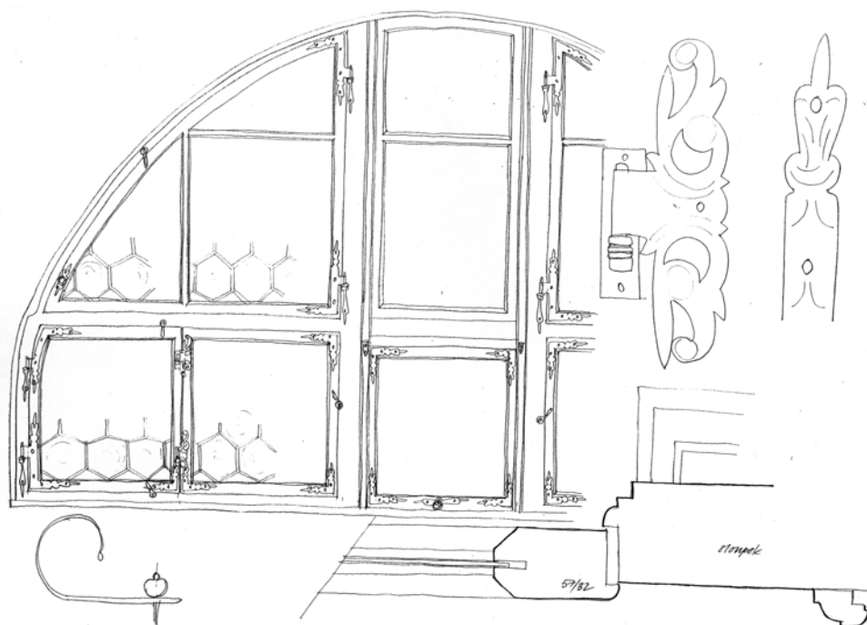
Obr. 5: Zásnuky (okres Kolín), františkánský klášter, oratoř kostela, okno s výsuvným středním spodním křídlem. (Skica J. Mrázek)
