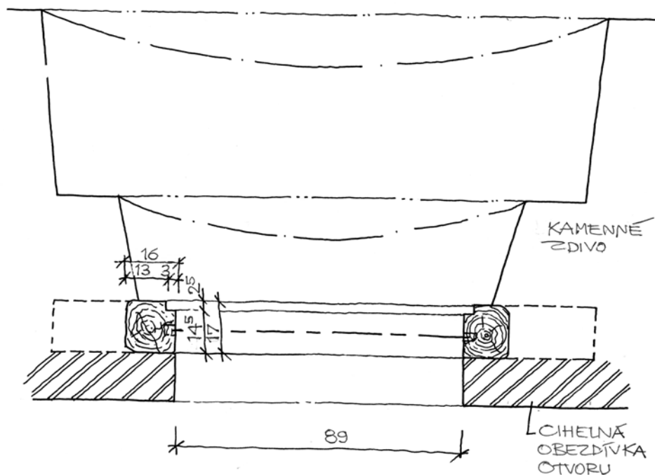
Obr. 1: Třebešice (okres Benešov), zámek, přízemí, jižní fasáda, půdorysný řez trámkovou zárubní okenního otvoru. Podle zjištění Jana Veselého jde zřejmě o pozůstatek okna starší tvrze. (Skica J. Veselý)
