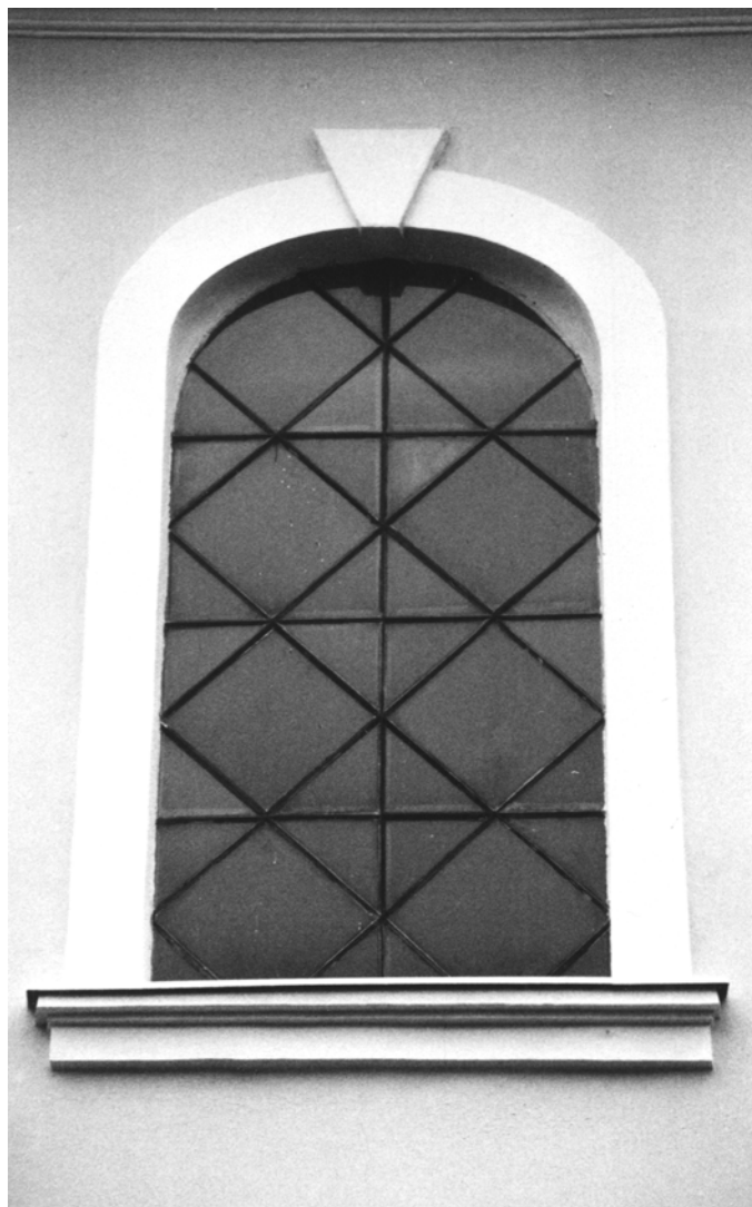
Obr. 8: Sedlčany (okres Příbram), kostel Nanebevzetí P. Marie, lod', okno jižní fasády. (foto autor) Subtilní ocelové pruty t.zv. okenního profilu, známé rovněž pod názvem Fenestra, nebyly využívány jen u průmyslových a hospodářských staveb. Jsou hlavním konstrukčním materiálem mnoha chrámových oken. Některá z nich jsou členěna pouze ortogonálně, u jiných bylo realizováno výraznější architektonické řešení. Ani těmto oknům nelze upřít určitou památkovou hodnotu.
