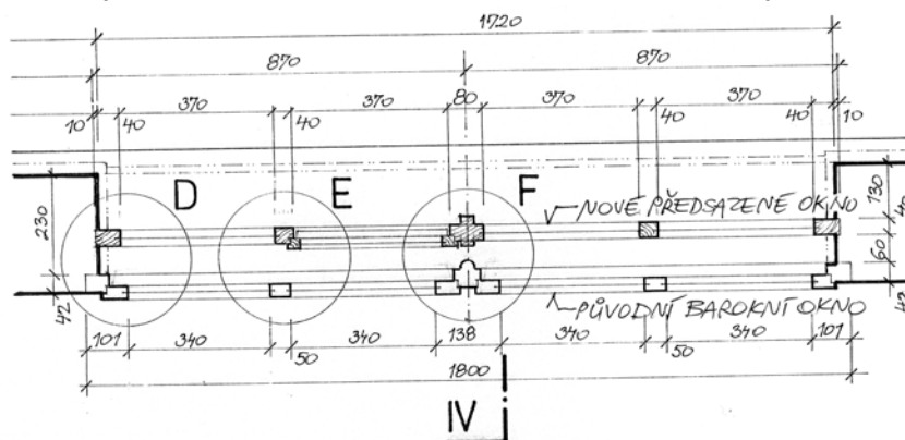
Obr. 13: Slaný (okres Kladno), františkánský klášter, ambit, půdorysný řez okenním otvorem. (Kresba J. Adámek)
