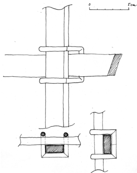
Obr. 3: Kozmice (okres Benešov), kostel sv. Jakuba Většího, presbytář, gotické okno východní fasády. Detail křížení původního vodorovného kovaného pásu s dodatečně přidaným svislým pásem. (Skica J. Veselý)
