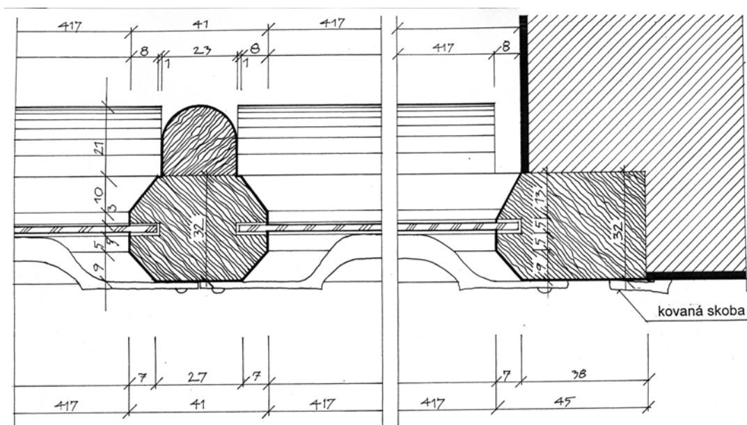
Obr. 4: Nabdín (okres Kladno), kostel Sv. Barbory, loď, severní průčelí, vodorovný řez sloupkem a zabudovaným rámem okna. (Kresba M. Prchal)
